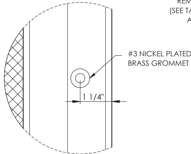
4 10 GROMMET - DETAIL N.T.S.
